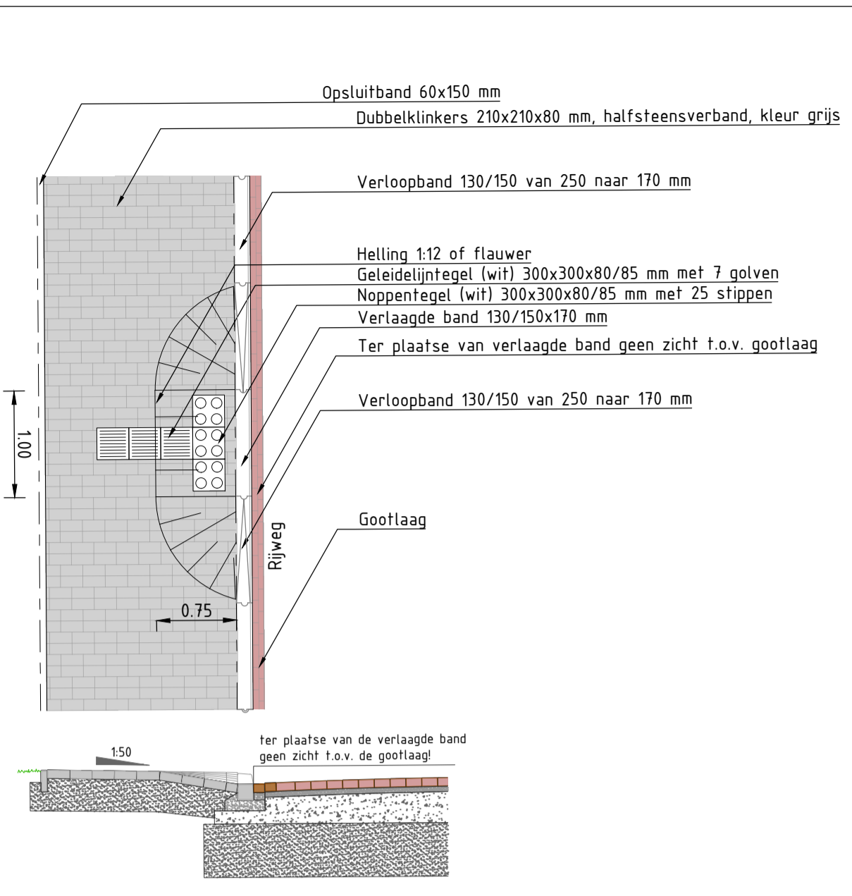
Principedetail mindervaliden oversteekplaats Schaal 1:50
