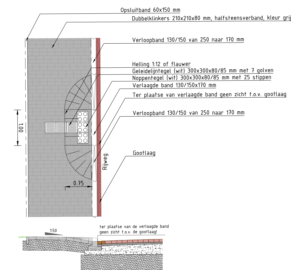
Principedetail mindervaliden oversteekplaats
